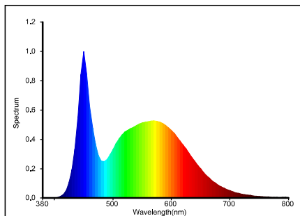
E5 DL03 25W 6000K
