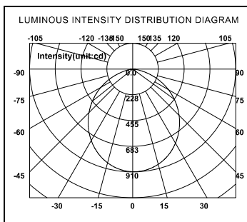
E5 DL03 18W 3000K
