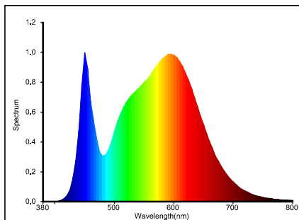
E5 DL03 25W 4000K
