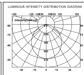
E5 DL03 25W 3000K
