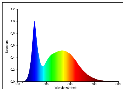
E5 DL03 15W 6000K
