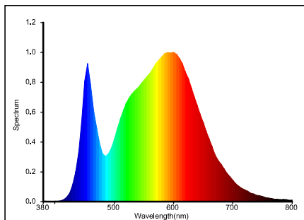
E5 DL03 18W 4000K
