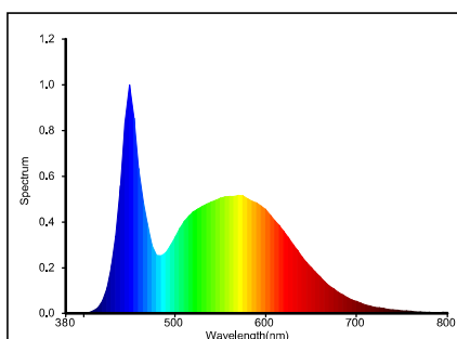
E5 DL03 18W 6000K
